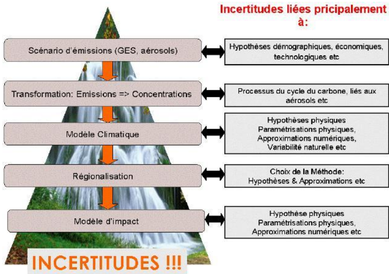
FIG. 3.7: La cascade des incertitudes caractéristique d'une étude des impacts du changement climatique
